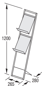
P-2 2 DIN A4- Ablagen
