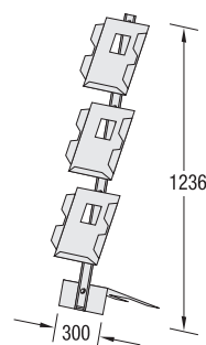
PL-3 3 DIN A4-Ablagen aus Lochblech
