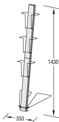
PG-3 3 DIN A4- Gitterkörbe
