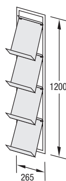
P-4W 4 DIN A4-Ablagen für Wandbefestigung
