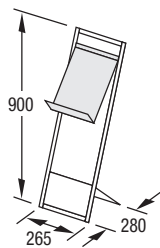
P-1 1 DIN A4- Ablage
