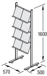
P-8 8 DIN A4- Ablagen
