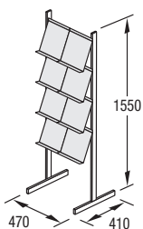
P-8L 8 DIN A4- Ablagen
