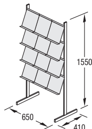
P-12L 12 DIN A4- Ablagen
