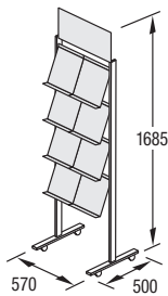
P-8T 8 DIN A4-Ablagen + Topschild
