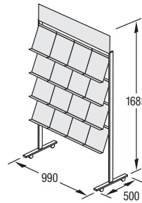
P-16T 16 DIN A4-Ablagen + Topschild
