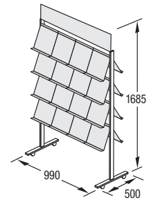
P-32T 32 DIN A4-Ablagen + Topschild
