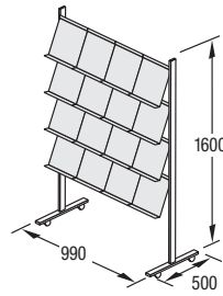
P-16 16 DIN A4- Ablagen
