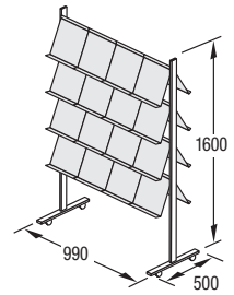
P-32 32 DIN A4- Ablagen
