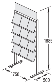
P-12T 12 DIN A4-Ablagen + Topschild
